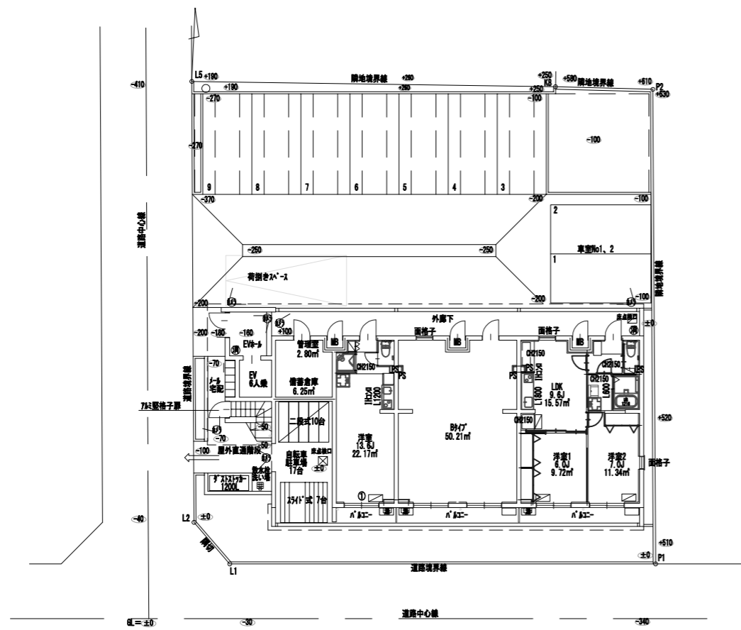
1階平面圖
